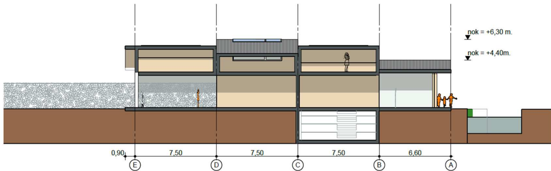
langsdoorsnede
