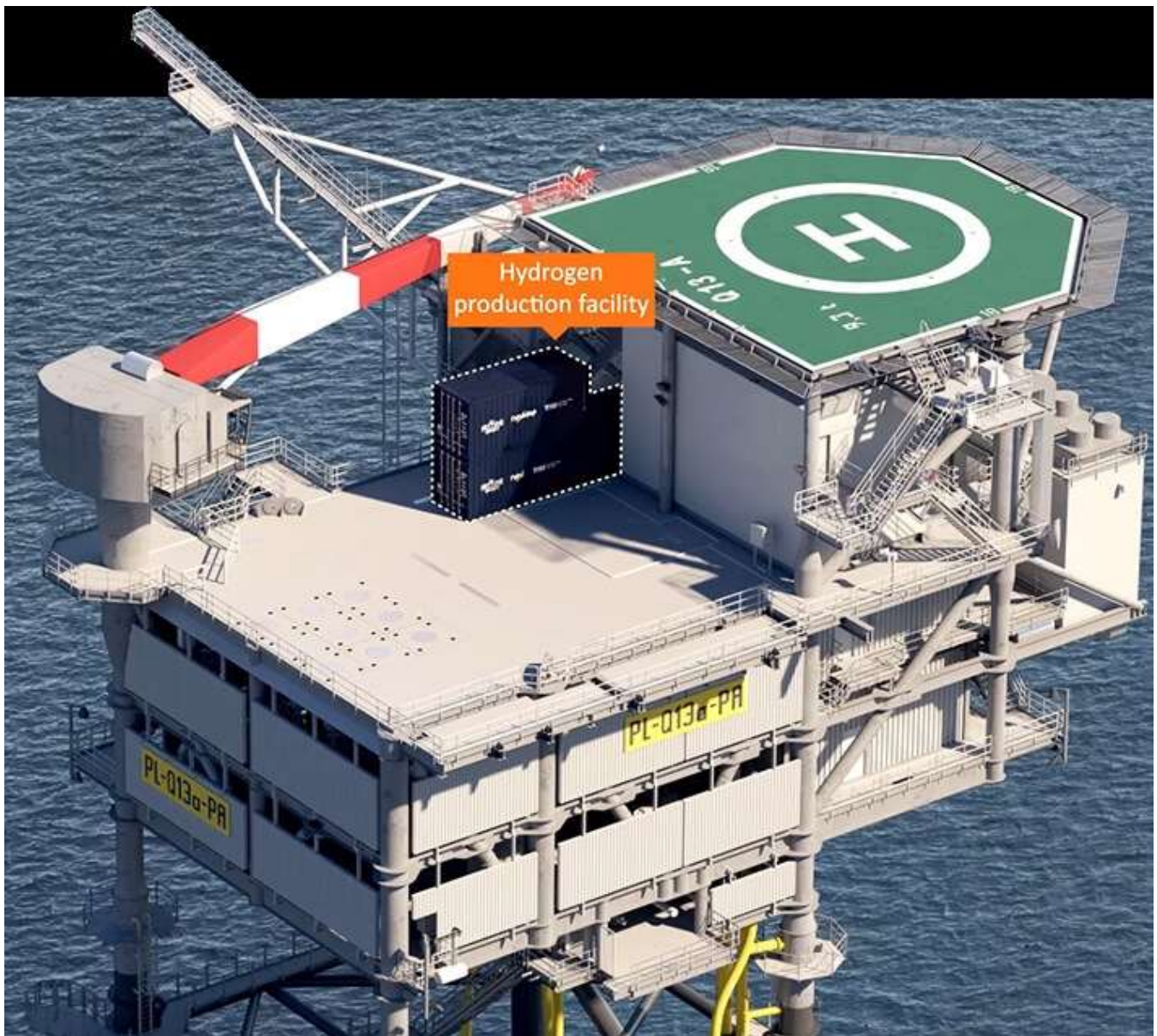
PosHYdon installatie: groene waterstof uit zeewater.
